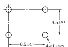
端子配置/内部连接图 (TOP VIEW)
