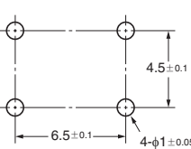
端子配置/内部连接图 (TOP VIEW)
