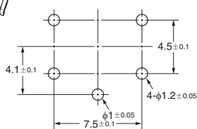
端子配置/内部连接图 (TOP VIEW)
