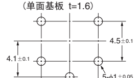
印刷基板孔加工尺寸示例 (TOP VIEW) (单面基板 t=1.6)
