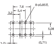
印刷基板加工尺寸 (BOTTOM VIEW) 尺寸公差±0.1mm
